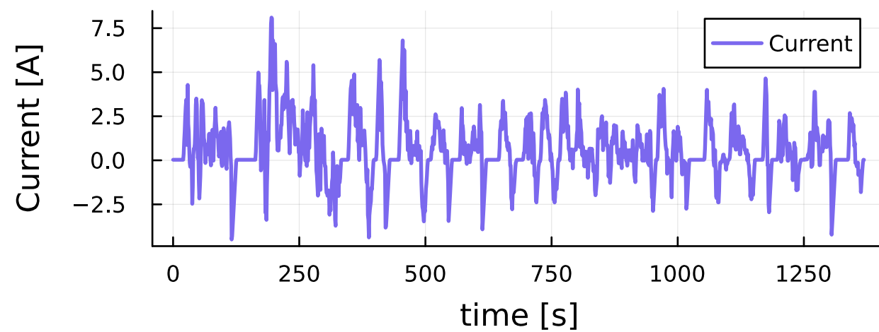
UDDS Current Profile
